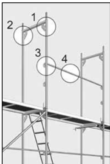
Overzicht aanhaakpunten
